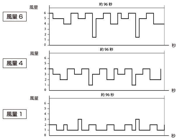
風量設定(例)
